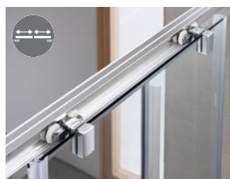
Rodamiento superior
